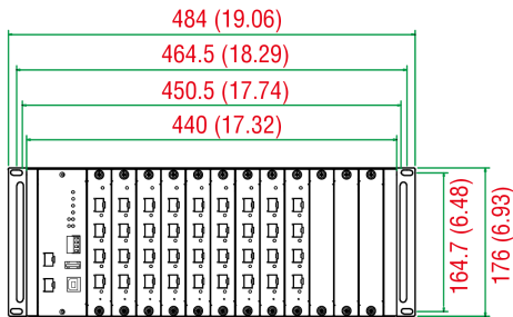
前视图
