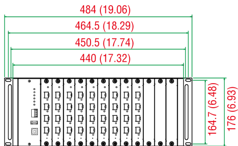
主视图
