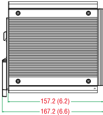
侧视图
