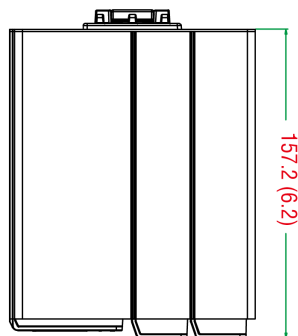
俯视图
