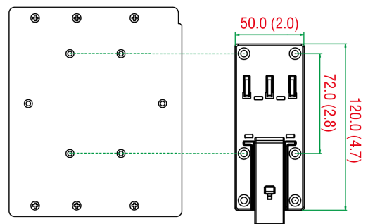
后视图
