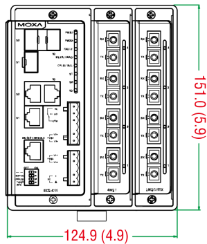
前视图
