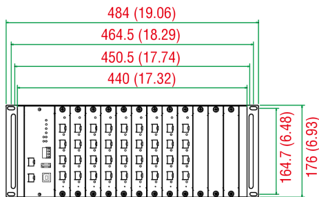
前视图
